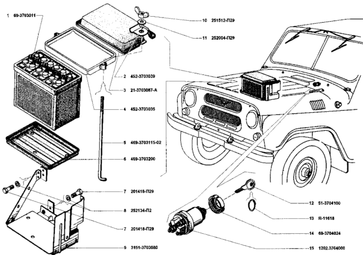
Kuva 90: Akku, virtalukko
